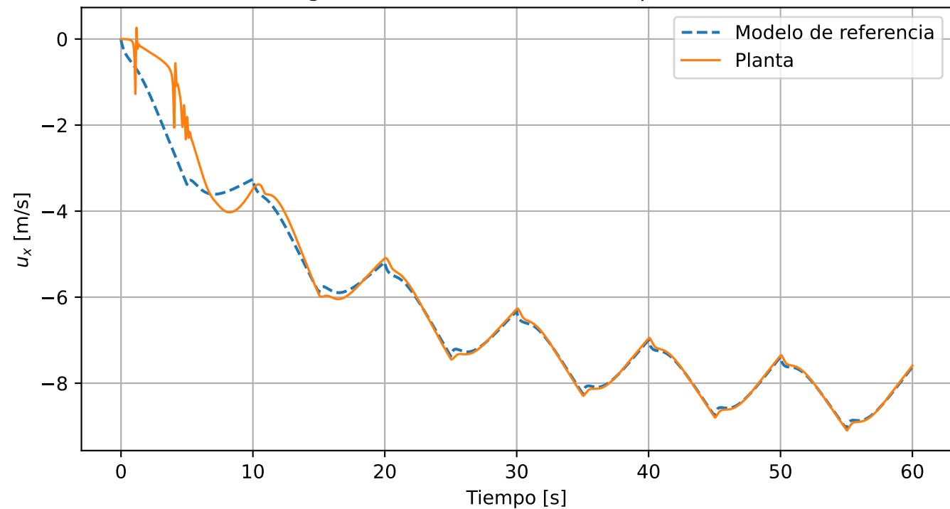
Seguimiento MRAC con tren de pulsos: u_x
